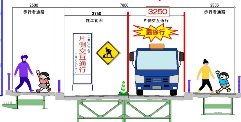
断面図
